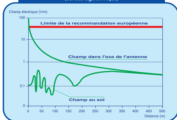
Champ reçu en fonction de la distance (échelle logarithmique)
