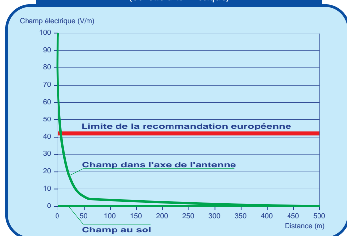
Champ reçu en fonction de la distance (échelle arithmétique)
